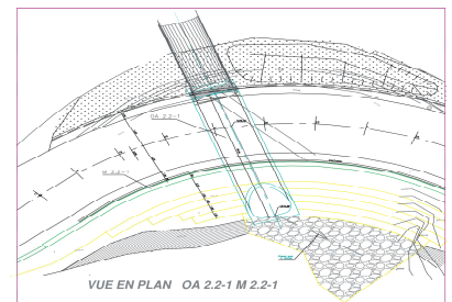
Vue en plan avec recalibrage du rayon routier
